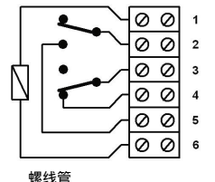
DPST-双刀单掷 NC+NO
